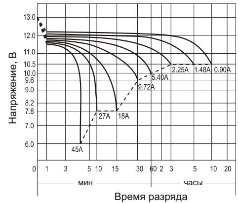
Разрядные характеристики
